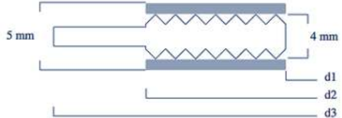
Kammprofilichtung nach Werknorm 146 für Flansche gemäß ASME B16.5
